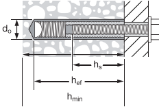
圖 8 — 喜利得 HIS-N 和 HIS-RN 規範
