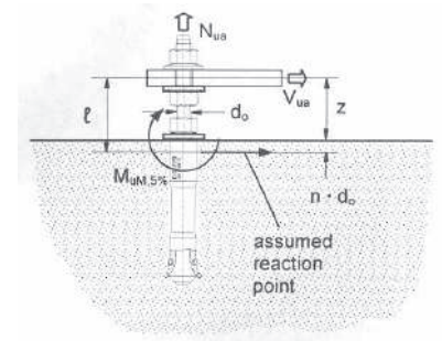
螺栓彎曲測定 — 強度設計
