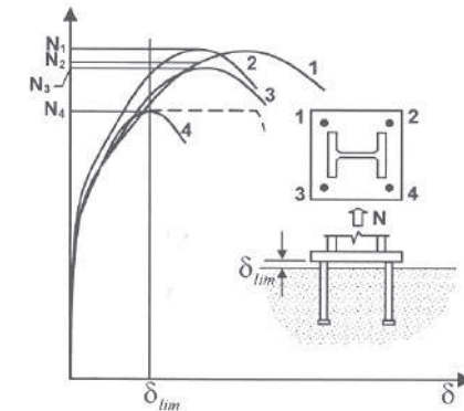
變形 (位移) 不相容性範圍
