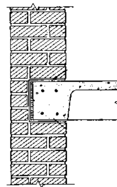
305mm 承重磚牆
