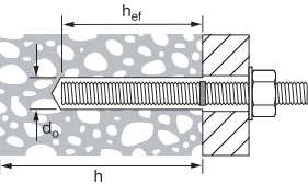
圖 1 — 喜利得 HAS-U-T(-R2) 螺桿
