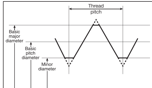
圖 1 - 螺絲螺紋的基本外形
