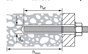
圖 10 — 喜利得 HAS-U-T(-R2) 螺桿
