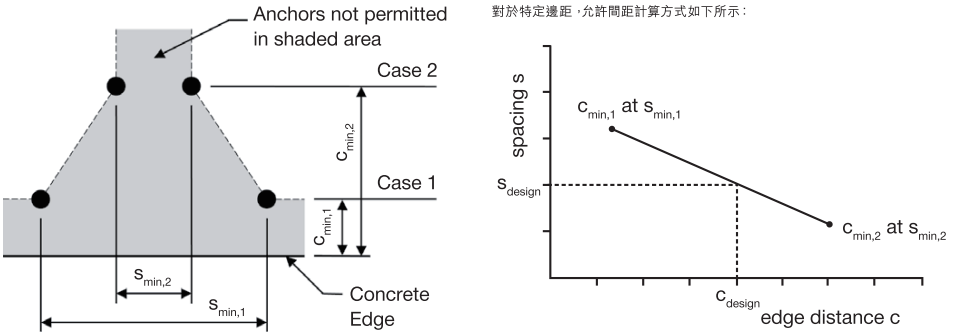
圖 5 — 最小邊距和錨栓間距的內插法
