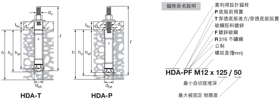
圖 1 — 喜利得 HDA 規格
