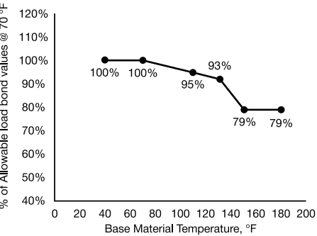
圖 14 — 溫度對於黏結強度的影響 1
