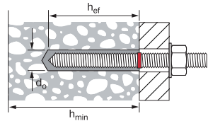
圖 2 — 使用喜利得 HVU2 錨栓膠囊安裝的喜利得 HAS-U-T(R2) 螺桿
