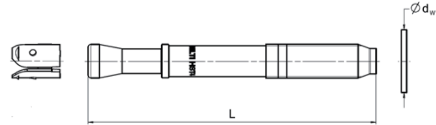
HST4(-R) M20
