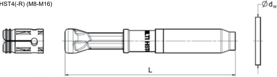
HST4(-R) (M8-M16)
