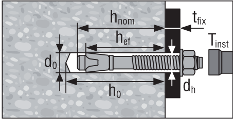
圖 1 — 喜利得 HST4 規格
