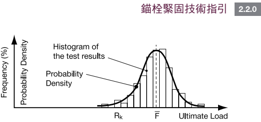
圖 2.2.1 錨栓極限荷載的頻率分布，顯示 5% 分位數的顯著性
