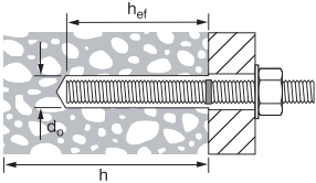
圖 4 — 喜利得 HAS-U-T(R2) 螺桿
