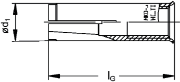
錨栓主體
