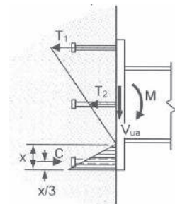
樑牆連接的彈性荷載分佈範例
