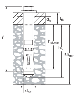
圖 1 — 安裝條件中的 HSL-3-R 和 HSL-3-GR (顯示 HSL-3-R)
